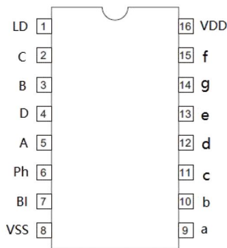
DIP-16/SOP-16/TSSOP-16
