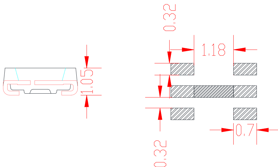
建议焊盘尺寸
