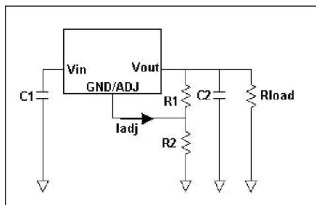
图 2 XBLW AMS1117 可调型应用电路
