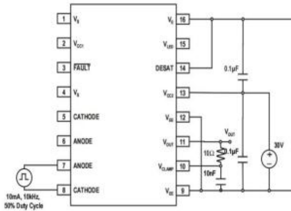
Fig 29. T_{PLH} , T_{PHL} , T_f , T_r Test Circuit
