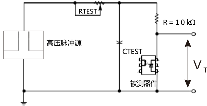
Fig.7 静态 dv/dt 测试电路和波形 Static dv/dt test circuit and waveform
