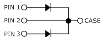
TO-247-3L
