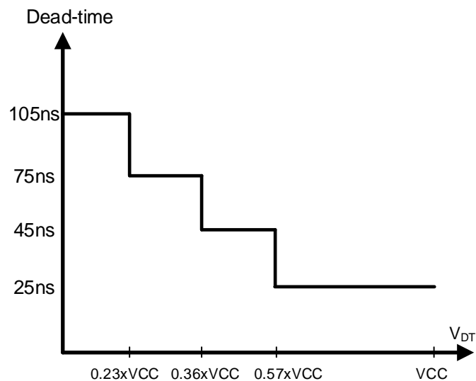
图 10-6 NSA2093 中死区时间与 V_{DT} 的关系
