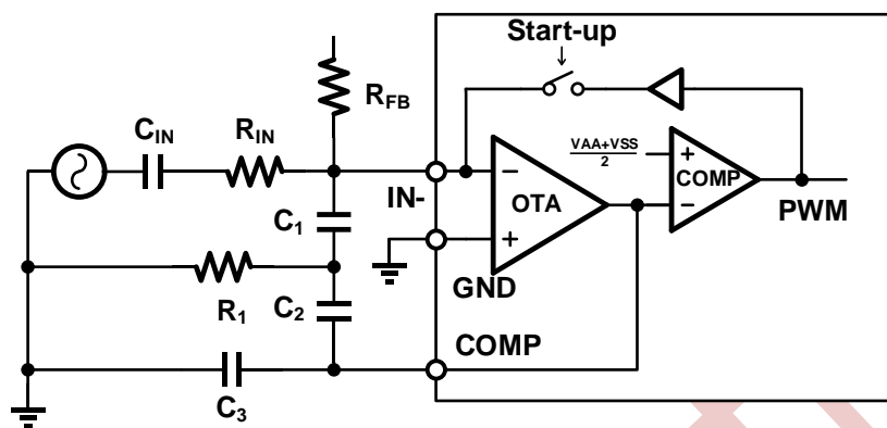
图 10-4 NSA2093 “咔哒” 噪声消除机制
