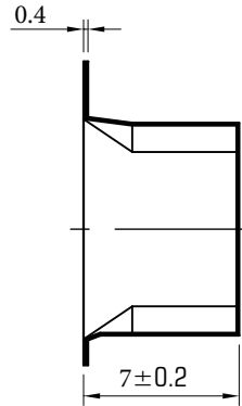
A-A剖面
