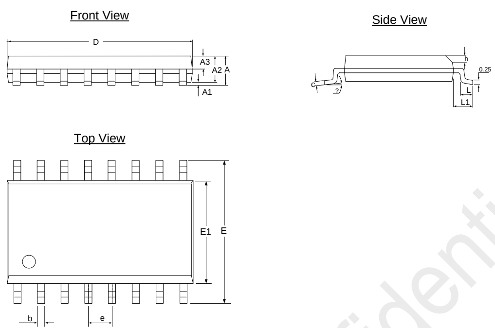
图 8. CMT810X SOIC-16 宽体封装
