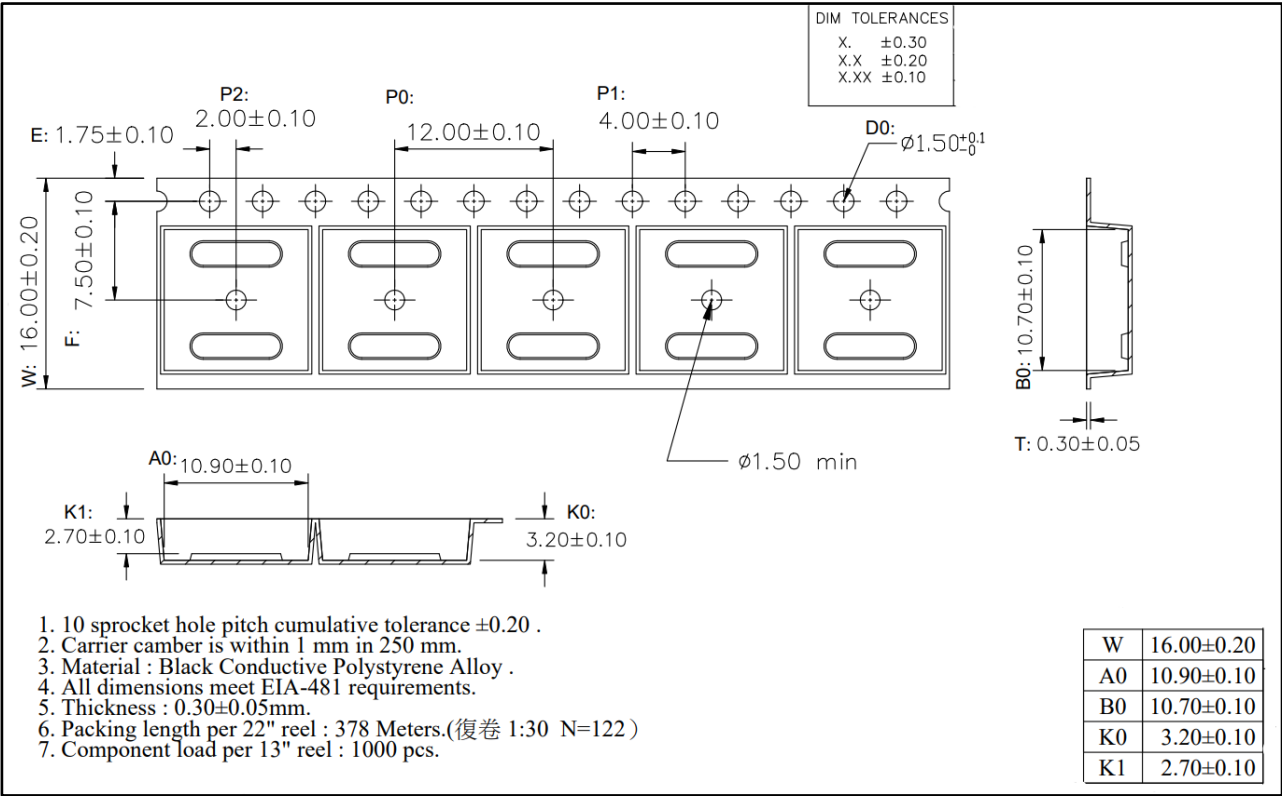
图 12. CMT810X WB SOIC-16 编带信息
