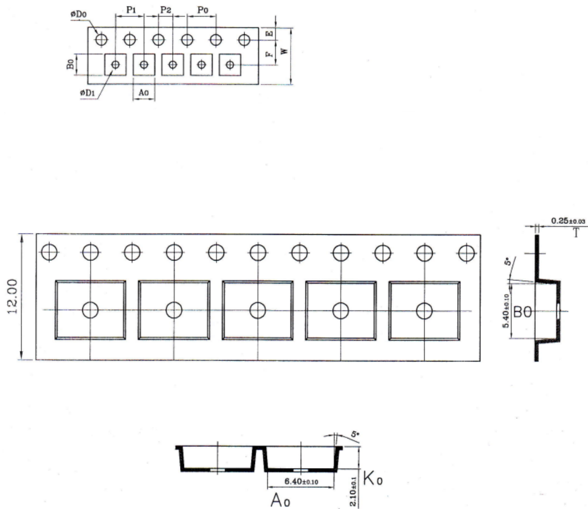
图 14.CMT810X NB SOIC-8 编带信息
