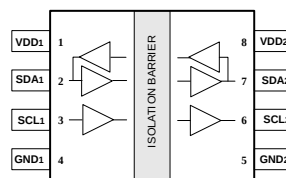
CMT8101N NB SOIC-8/ WB SOW-8
