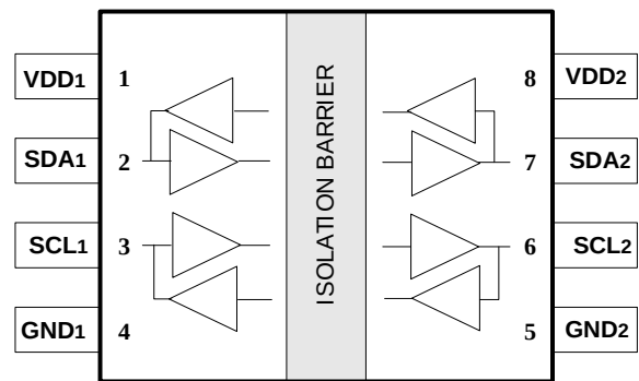
图 1. CMT8100N SOIC-8 窄体/SOW-8 宽体 管脚排列
