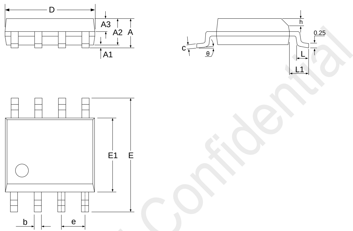
图 8. CMT810X SOIC-8 窄体封装
