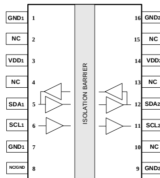
CMT8101W WB SOIC-16
