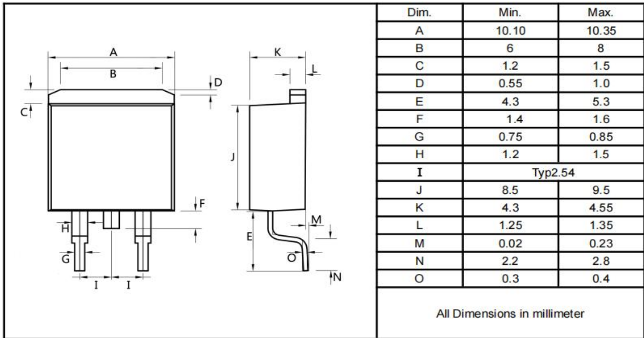
TO-263
