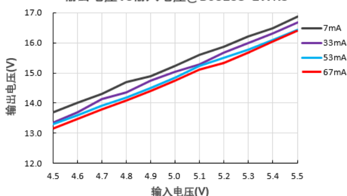
输出电压Vs输入电压@B0515S-1WR3
