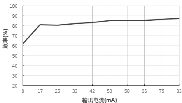
效率Vs输出电流(Vin=12V)@B1212S-1WR3
