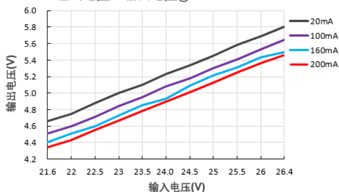
输出电压Vs输入电压@B2405S-1WR3
