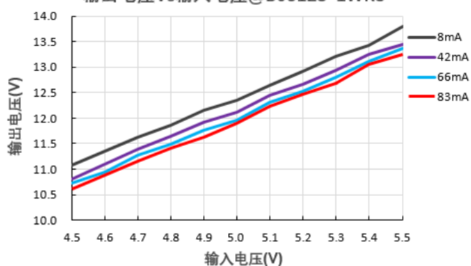
输出电压Vs输入电压@B0512S-1WR3
