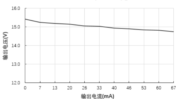
输出电压Vs输出电流(Vin=5V)@B0515S-1WR3
