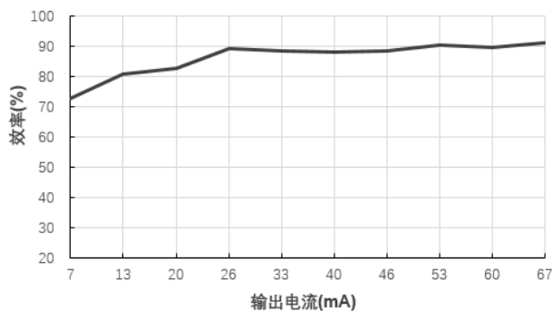
效率Vs输出电流(Vin=24V)@B2415S-1WR3
