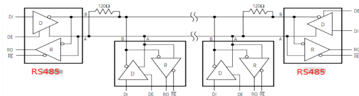
图 11 典型的 RS485 半双工通讯网络
