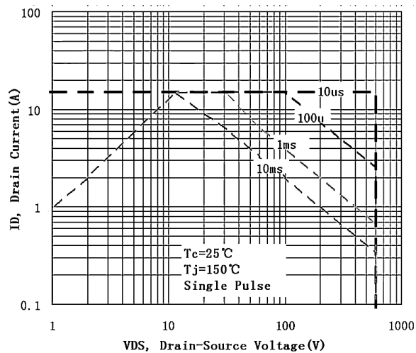
图 6-2 4N65(TO-220F)
