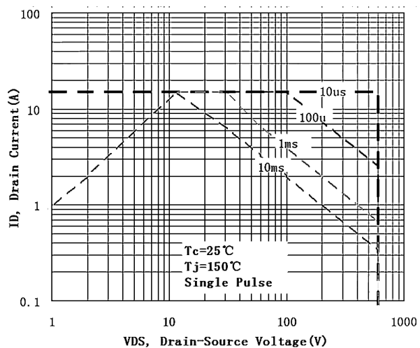
图 6-1 4N65(TO-220)
