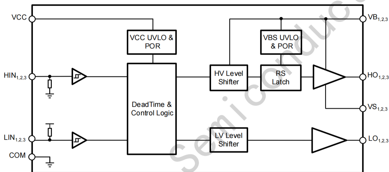
图 7-1 FD6288 功能框图
