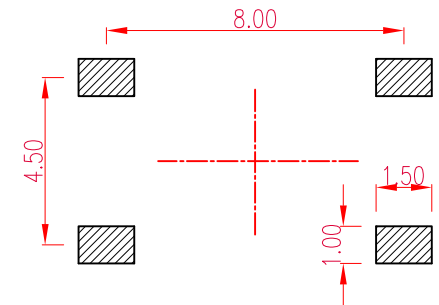
PCB. 焊接图
