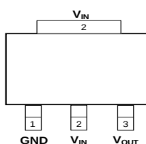
SOT89-3L(P1) Top View
