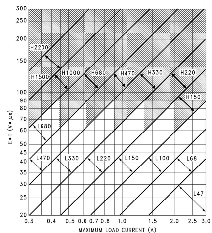
LM2576-ADJ
