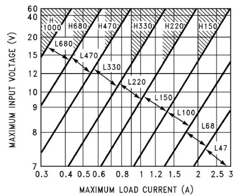
LM2576-5.0
