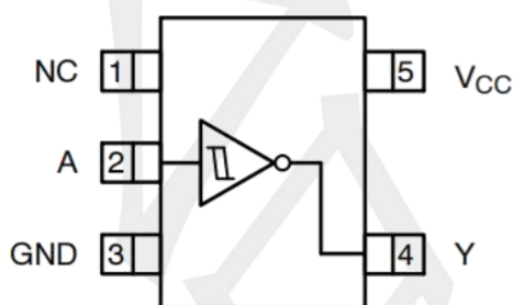
SOT353 / SOT23-5
