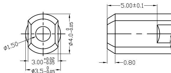
轴心部尺寸详图
