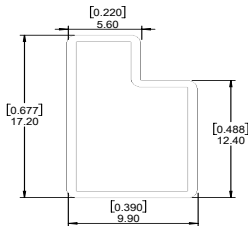
包装管尺寸图
