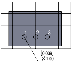
推荐 PCB 图
