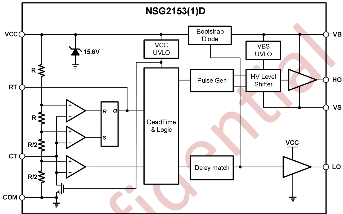
图 9-2 NSG2153(1)D 功能框图
