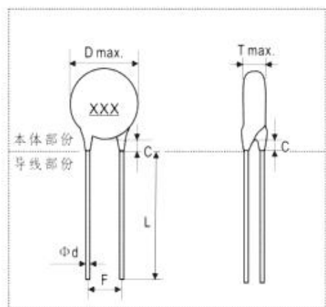
外形尺寸图
