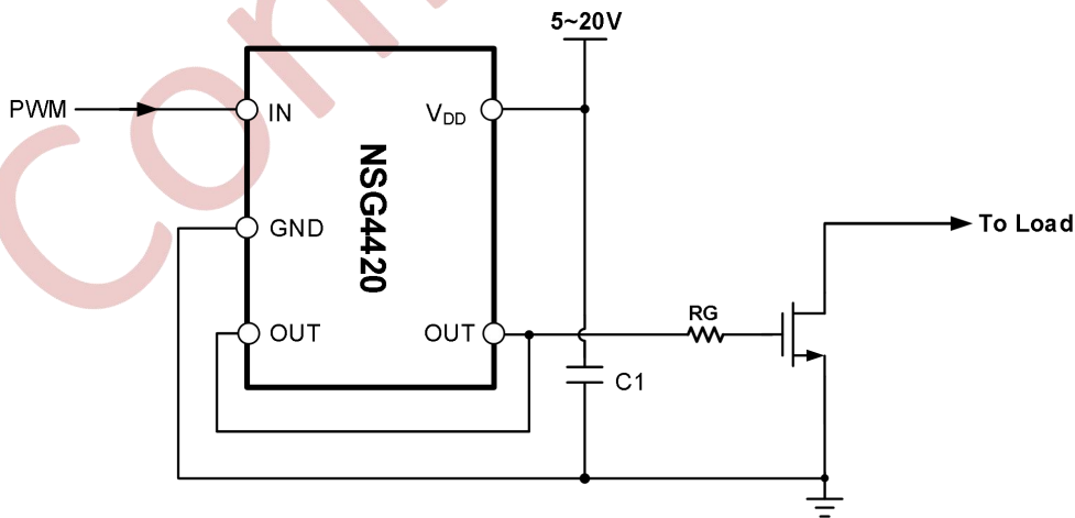
图 9-2 NSG4420 典型应用电路图
