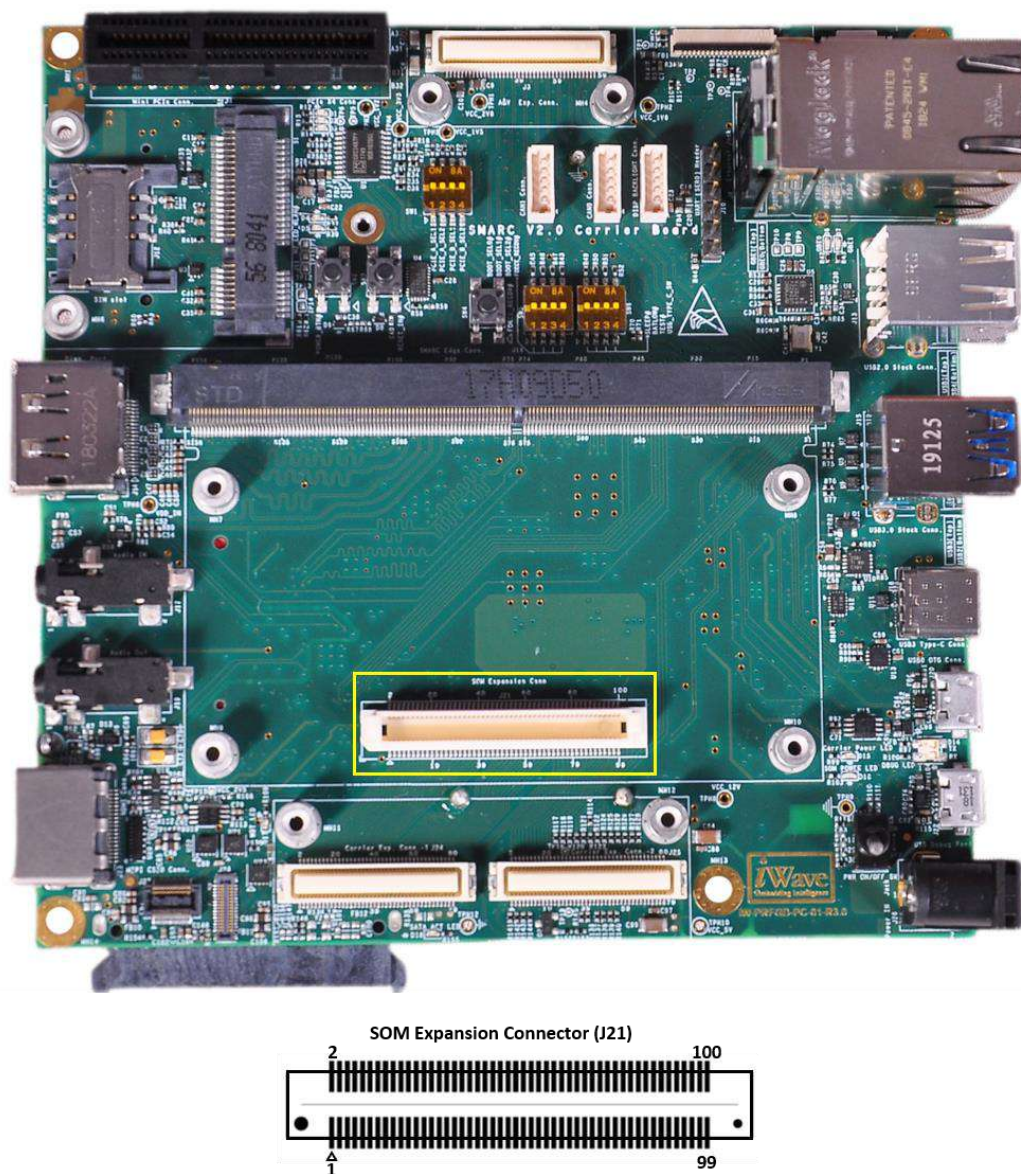
Figure 20: SMARC SOM Expansion Connector
