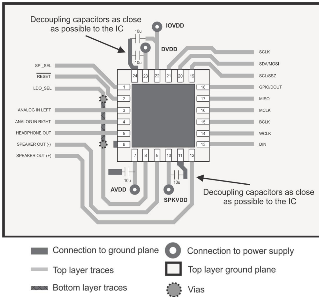
图 11-1. Layout Diagram
