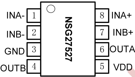
图 7-1 8-脚 SOP/WSOP 顶视图
