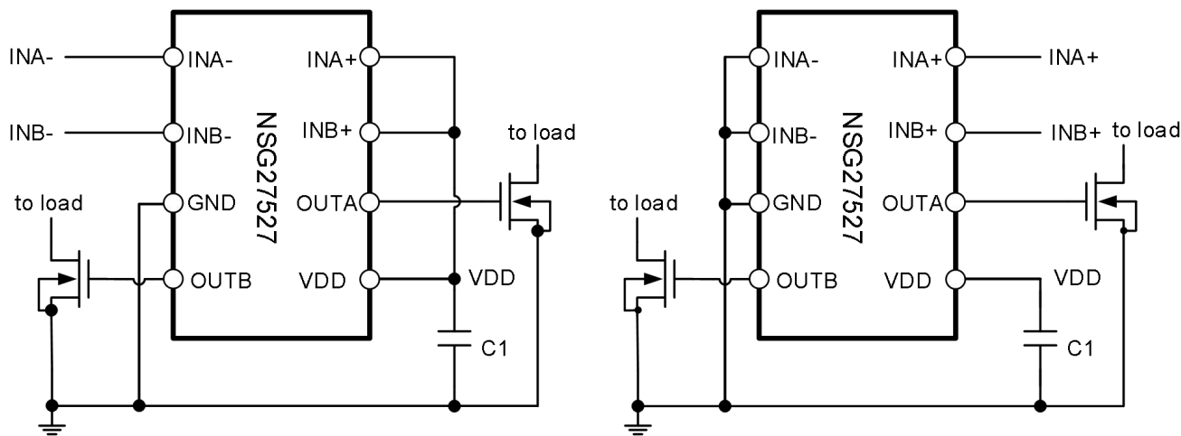
图 10-2 NSG27527 典型应用电路图
