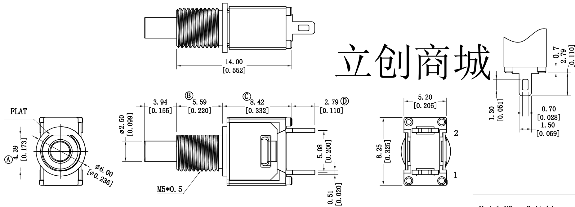
标注: ① - ④ 尺寸的重点检验尺寸
