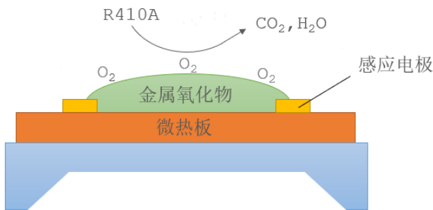
图 2. 原理示意图
