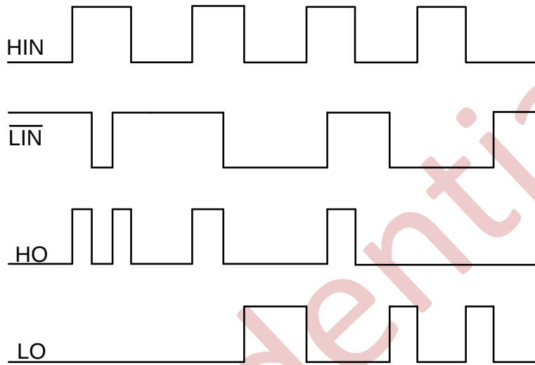
图 9-1 NSG6001 输入输出时序波形
