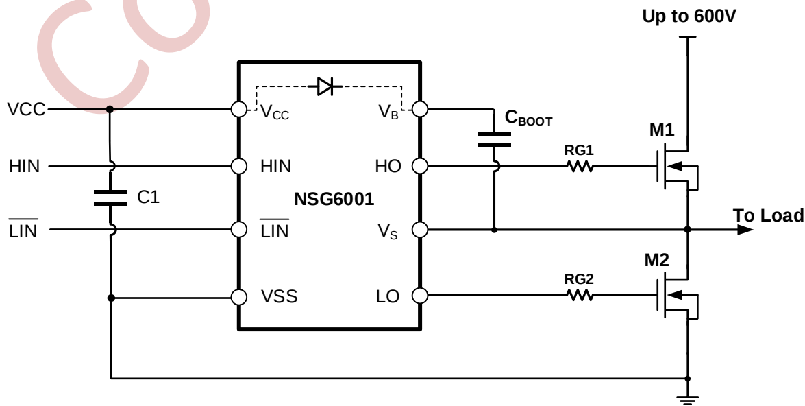
图 10-2 NSG6001 典型应用电路图
