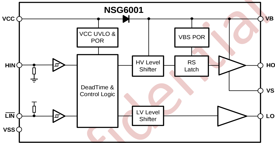
图 10-1 NSG6001 的功能框图
