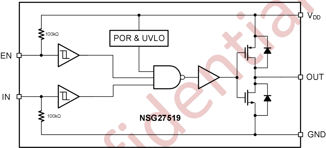
图 9-1 NSG27519 功能框图
