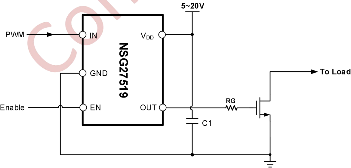
图 9-2 NSG27519 典型应用电路图
