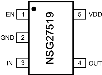
图 6-1 5 脚 SOT23-5 顶视图
