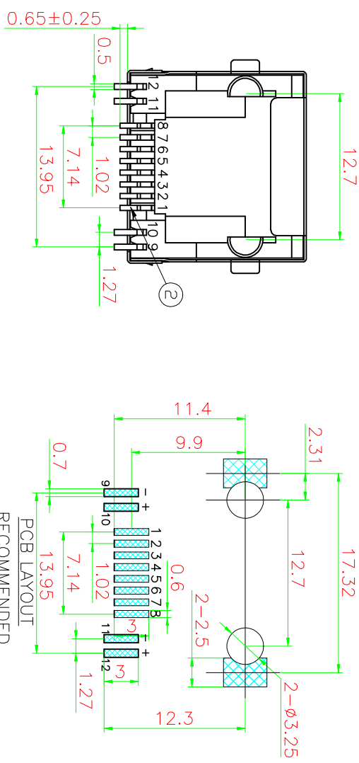
网络插座外形图
