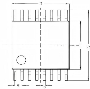
TOP VIEW 正视图
