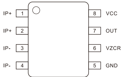
SOP8 Package
