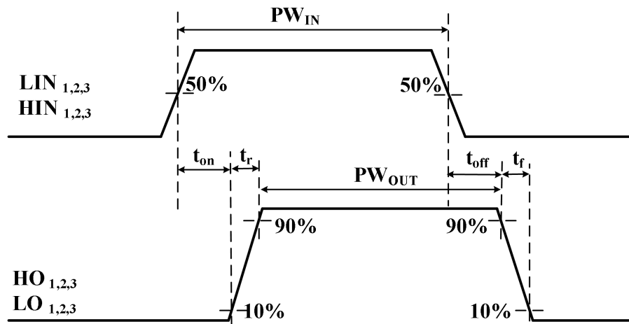
图 9-2 传输时间波形定义
