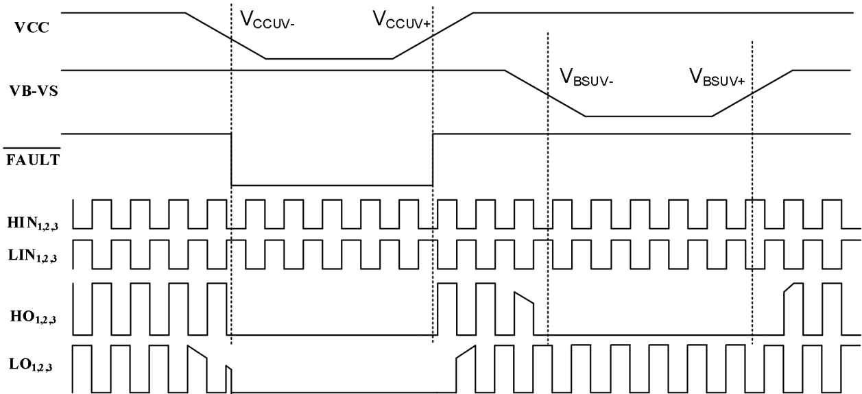
图 10-3 欠压功能波形定义
