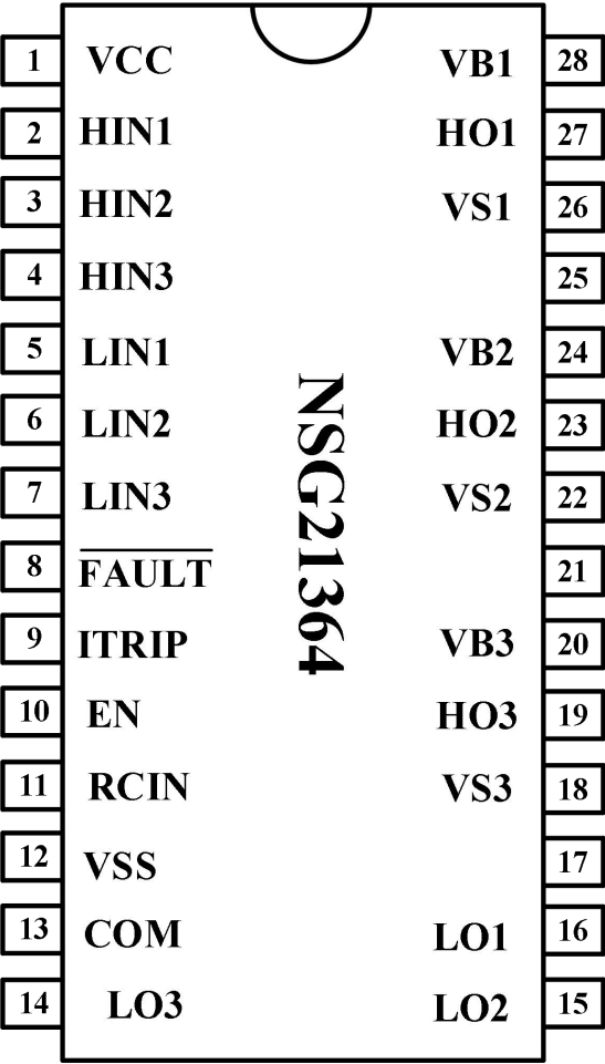
图 7-1 28-脚 SOP 顶视图
