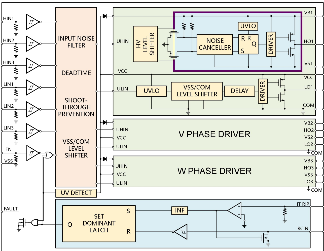
图 10-1 NSG21364 功能框图
