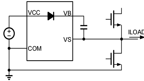
图 10-8 自举电路基本结构
