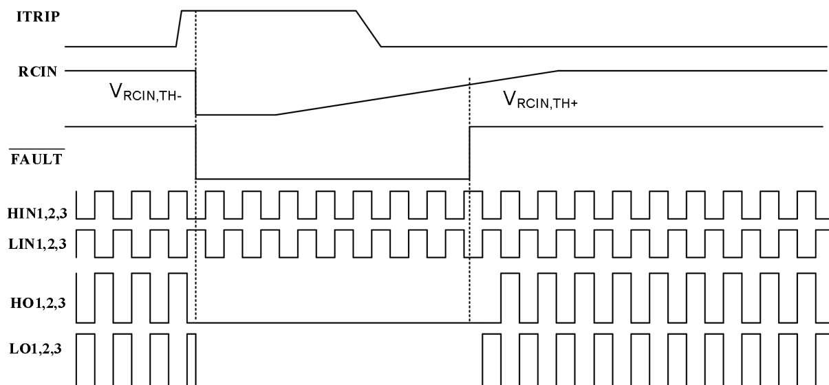
图 10-5 过流保护波形定义
