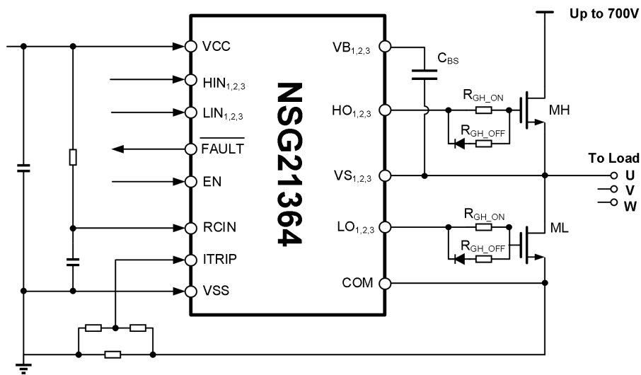
图 10-7 典型应用电路图
