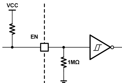
图 10-4 EN 引脚框图
