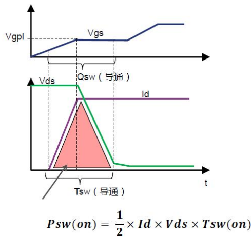
图 10-9 阻性负载条件下的 MOS 开关损耗
