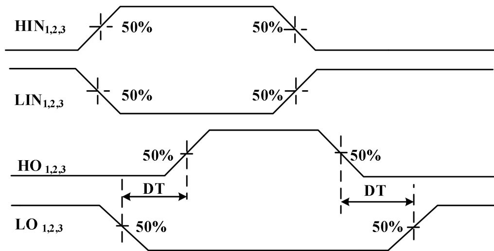
图 9-4 开关时间波形定义
