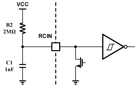
图 10-6 RCIN 引脚框图
