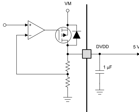
图 6-10. 线性稳压器方框图
