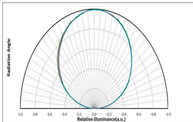
角度图, T_a=25^\circ\text{C}
