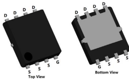
PDFN5X6-8L
