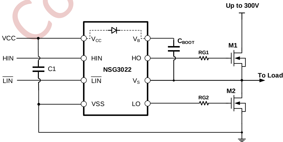
图 10-2 NSG3022 典型应用电路图
