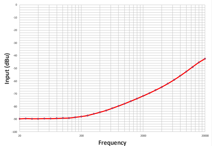
A-11J CMRR
