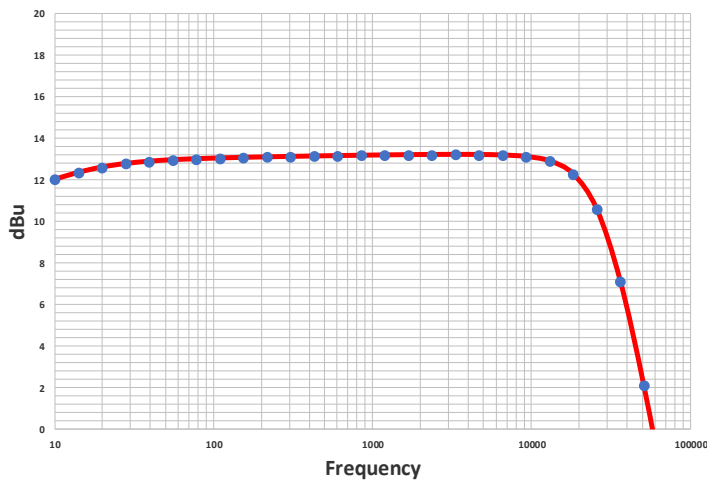
A-11J Amplitude
