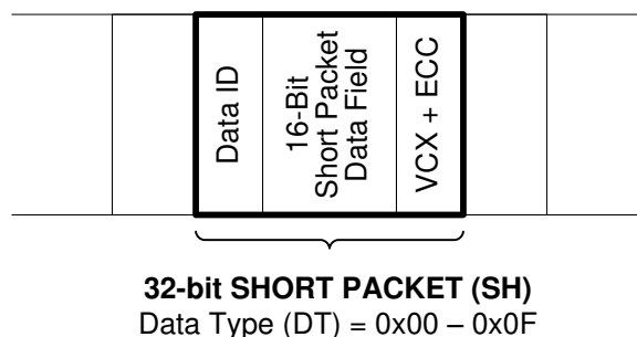
图 5-7. CSI-2 Short Packet Structure
