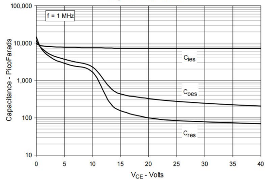
Fig. 10. Capacitance
