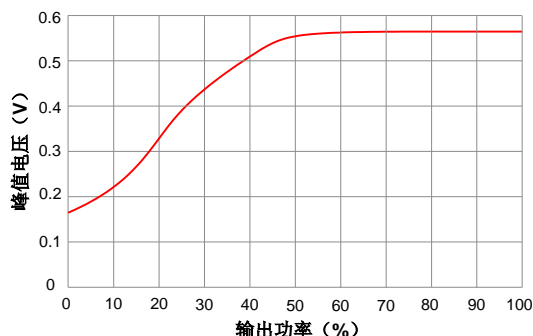
图 6. 峰值电流采样阈值
