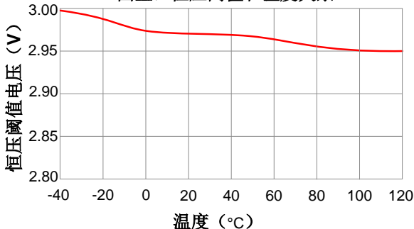
图五:恒压阈值和温度关系
