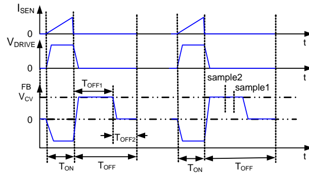
图 7. 恒流原理
