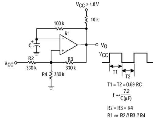
方波振荡器
