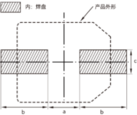
SMD推荐焊盘尺寸
