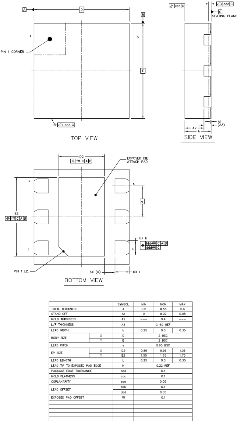
图 29. 6 引脚 DFN-6
