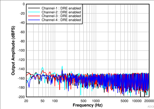
图 5-8. 空闲输入时的 FFT (DRE 已启用)
