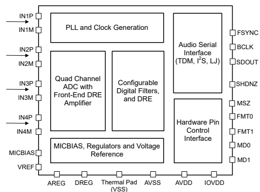
简化版方框图
