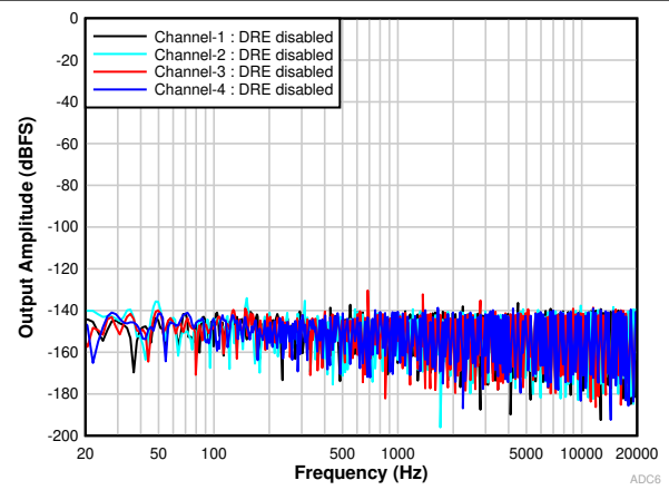
图 5-9. 空闲输入时的 FFT (DRE 已禁用)
