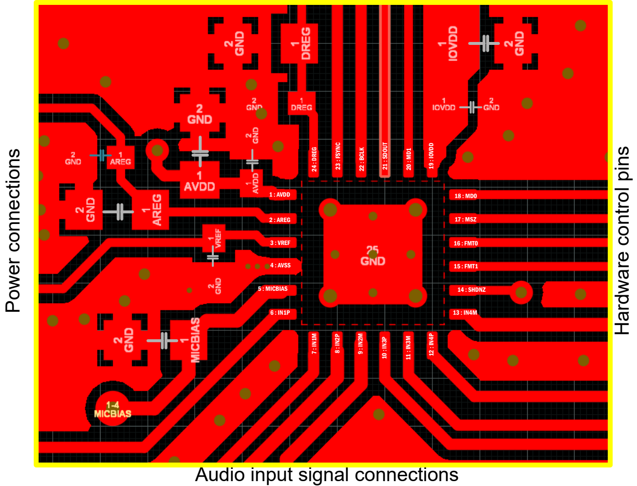
图 7-7. 示例布局
