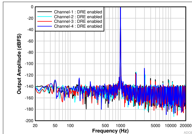
图 5-12. 具有 -1\text{dB} 输入的 FFT (DRE 已启用)
