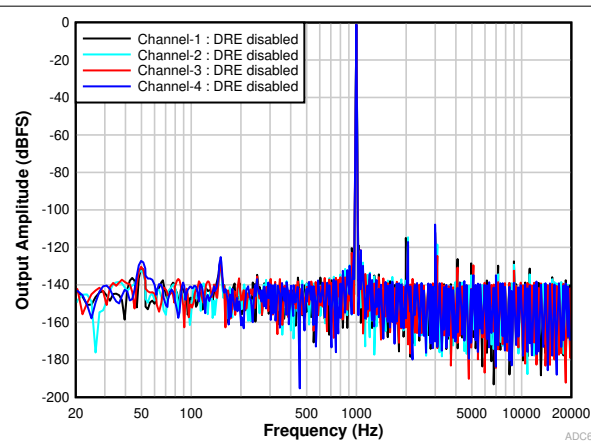
图 5-13. 具有 -1\text{dB} 输入的 FFT (DRE 已禁用)
