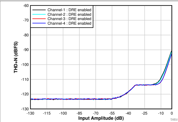
图 7-3. THD+N 与输入幅度间的关系 (DRE 已启用)
