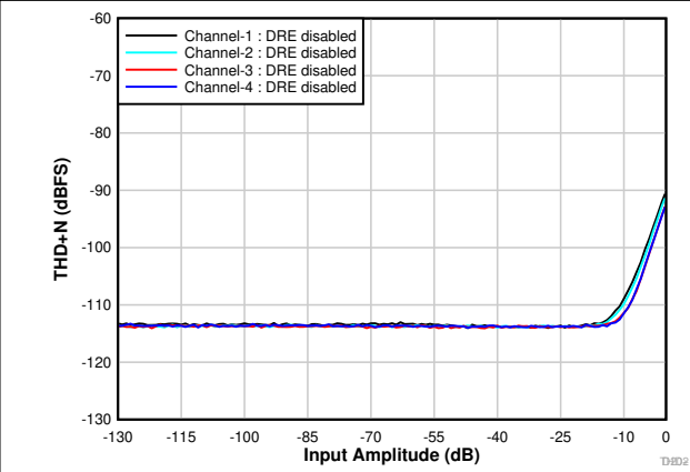
图 7-5. THD+N 与输入幅度间的关系 (DRE 已禁用)
