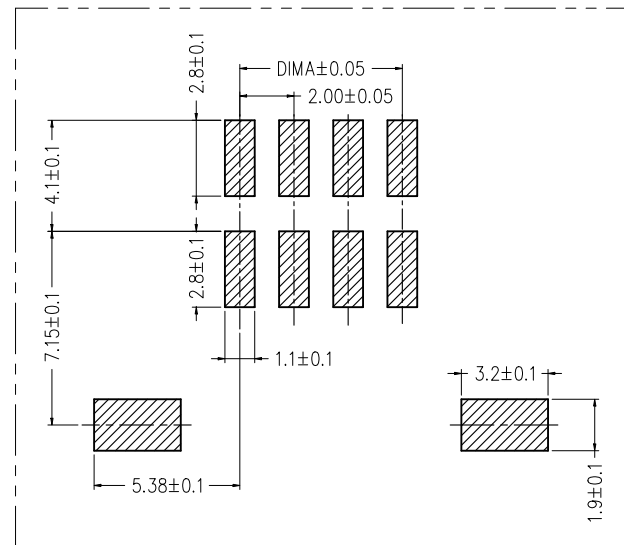
适用线路板 (PCB LAYOUT)
