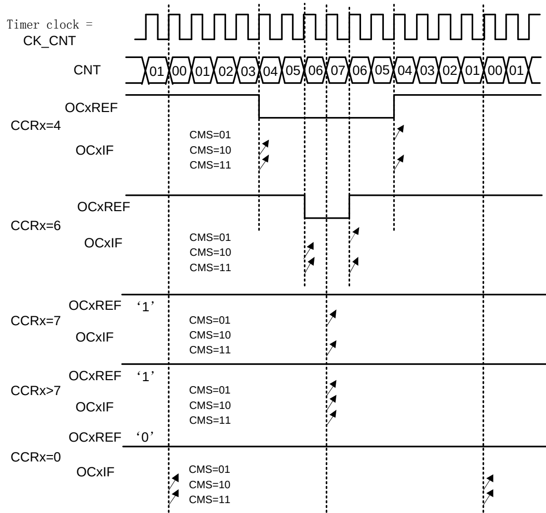
图28-29 中央对齐的PWM波形(APR=7)
