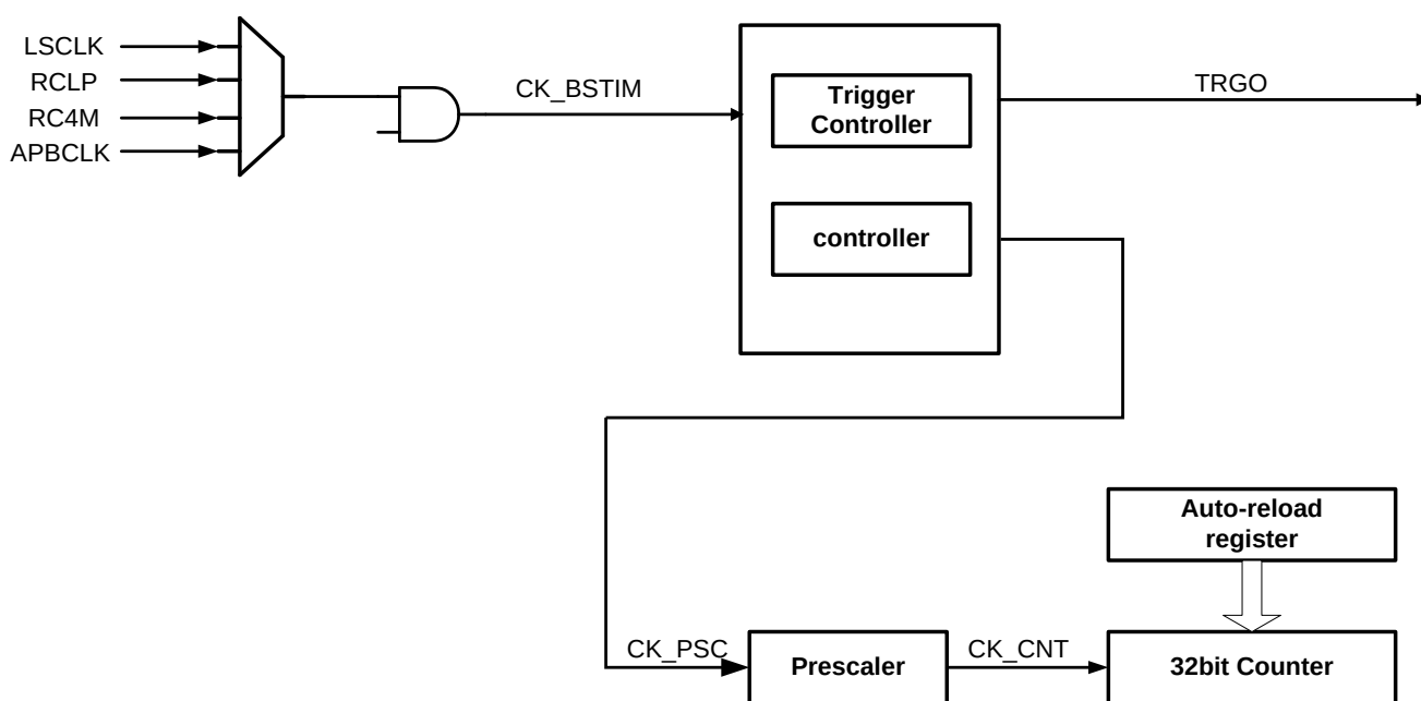
图29-1BSTIM32结构框图
