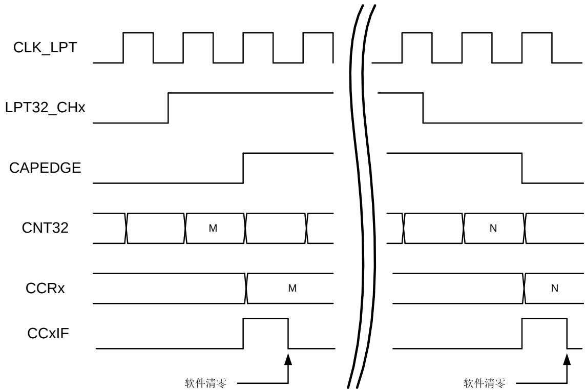
图 30-6PWM 输出
