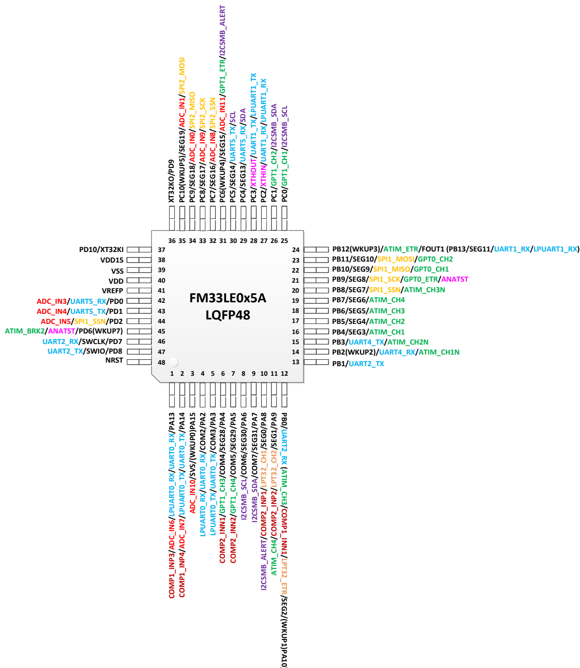
图 2-1FM33LE0x5A LQFP48 封装图
