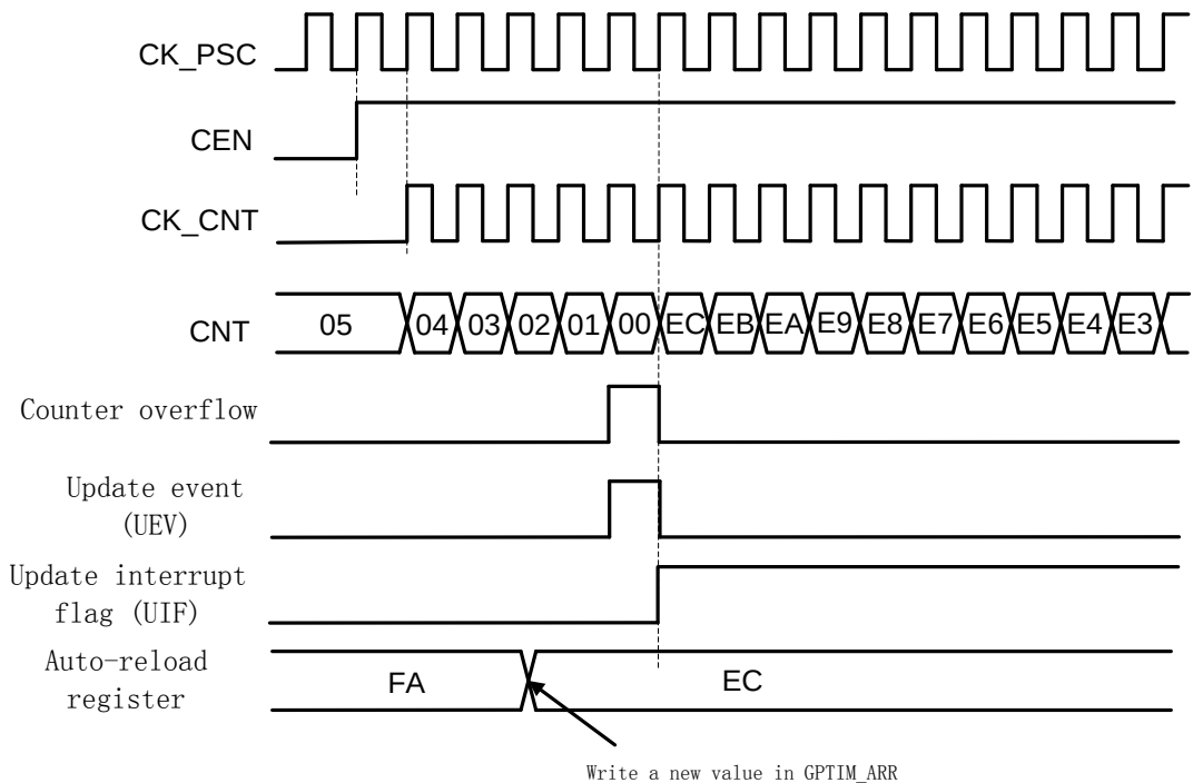
图 28-10 向下计数，内部时钟 2 分频
