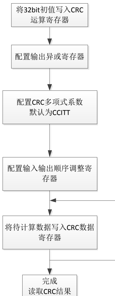
图 26-1CRC 运算流程图
