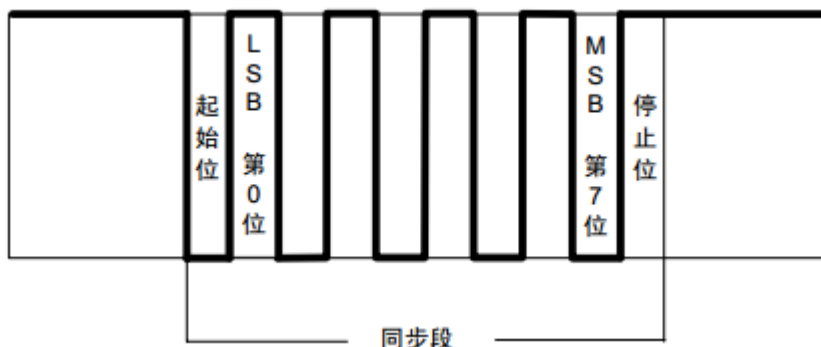
图 21-13 LIN sync field
