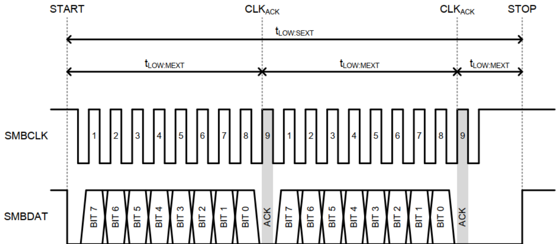
图 18-36 主机和从机超时事件
