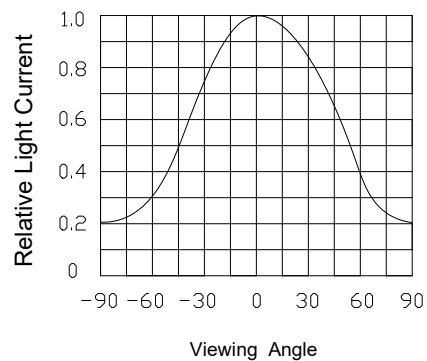
FIG.6 Angle VS Relative IL
