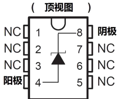
图 4 SOP8 管脚图
